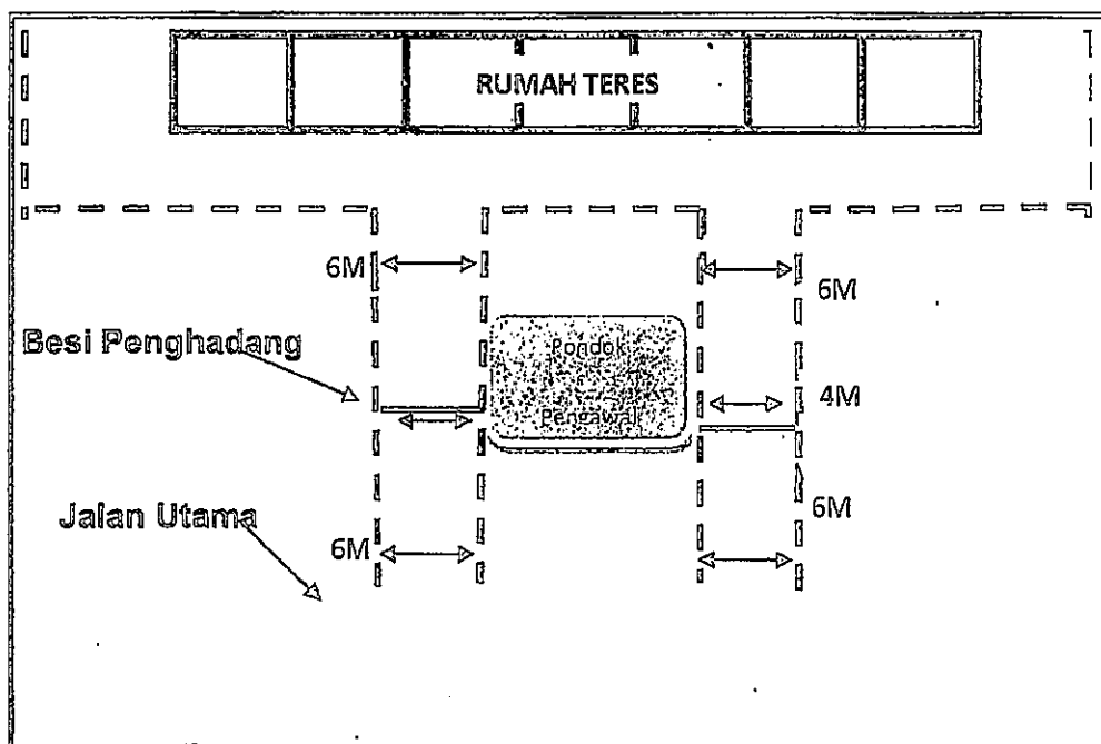
Rajah 5: Rajah menunjukkan bukaan kedua-dua pintu pagar minima adalah 4 meter.
